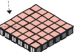
▲ Moduł światłoczuły Moduły pokrywają powierzchnię ogniskową o średnicy 2.26 m. Każdy z nich ma 6x6 = 36 fotonowielaczy (PMT) - elementów światłoczułych.
