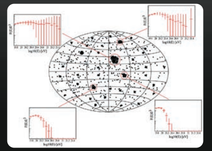
▲ Mapa nieba kierunków pochodzenia cząstek najwyższych energii, jakich możemy się spodziewać (1000 przypadków JEM-EUSO). Przypadki grupują się wokół kierunków wskazujących położenia silnych źródeł promieniowania kosmicznego najwyższych energii.
