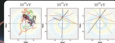
◀ Tory cząstek o niskich energiach są zakrzywiane i skręcane przez pola magnetyczne, ale cząstki powyżej 10^{20} eV poruszają się po trajektoriach prawie prostoliniowych, niemal niezmiennych przez pola magnetyczne. Tym samym zachowują one informację o kierunku ich pochodzenia.
